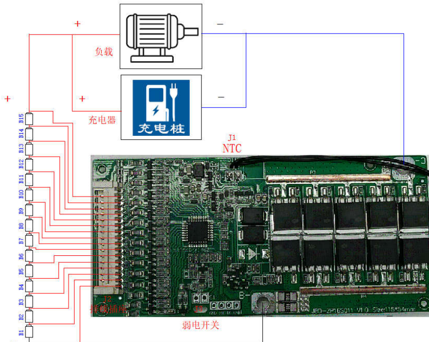
15 串接线示意图
