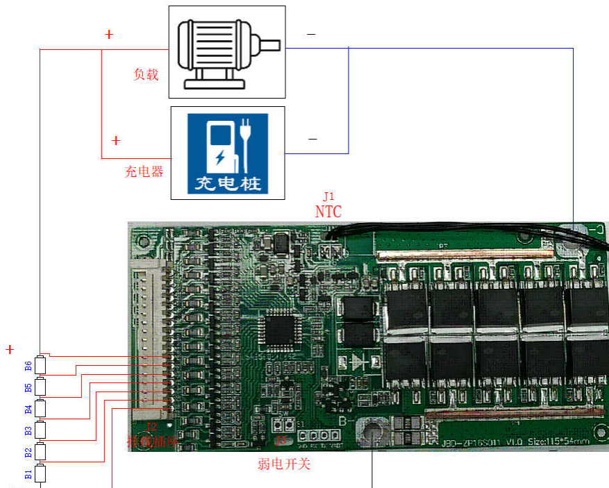
6 串接线示意图
