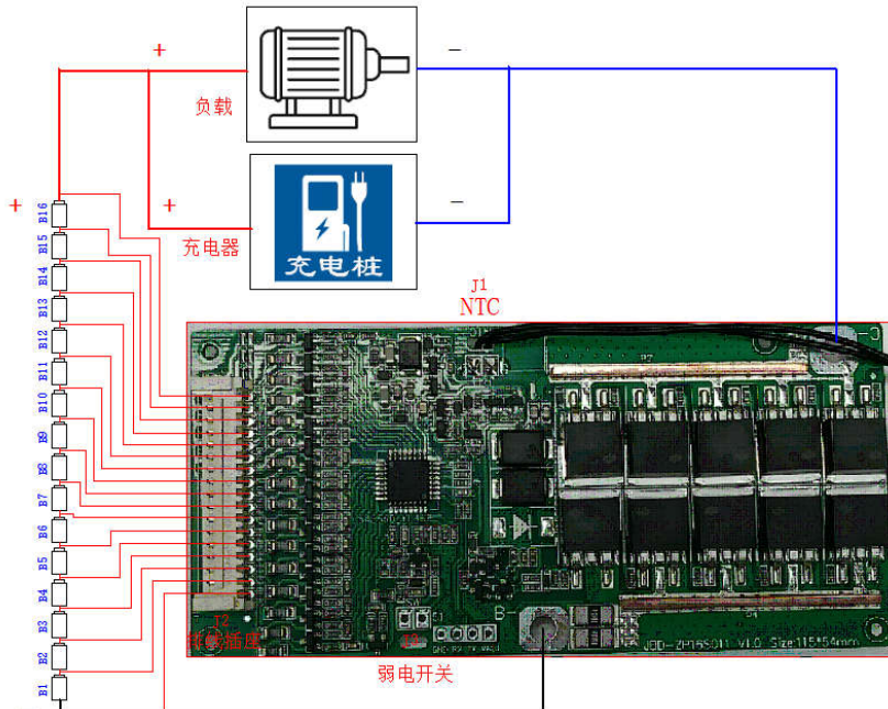
16 串接线示意图
