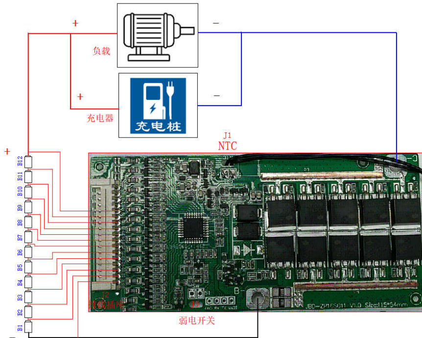
12 串接线示意图
